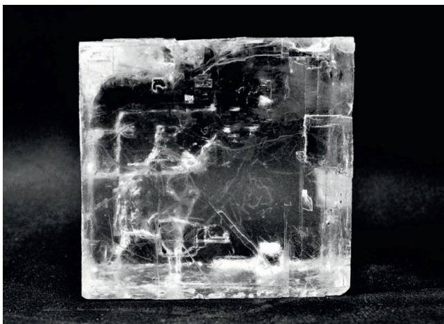
Кристал галіту з Артемівського родовища кам'яної солі. Фото Михайло Кулішов
